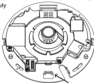
Obudowa kopuły
